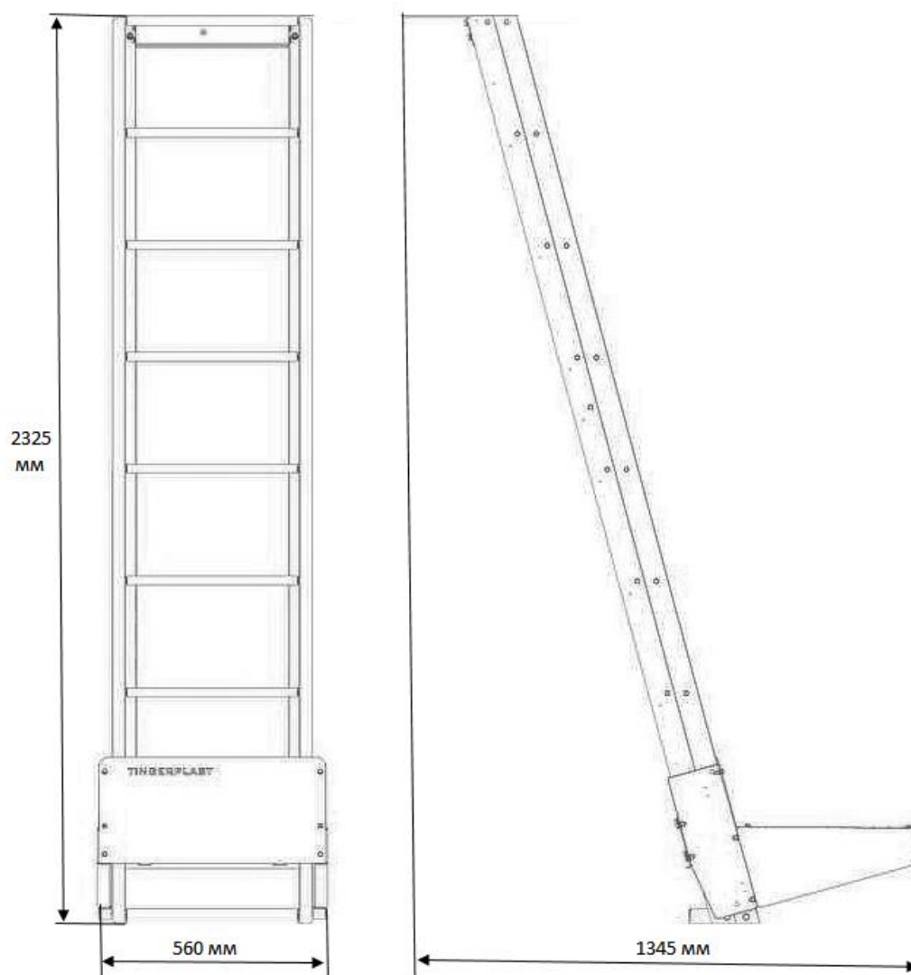
Рис.1. Размеры изделия.
